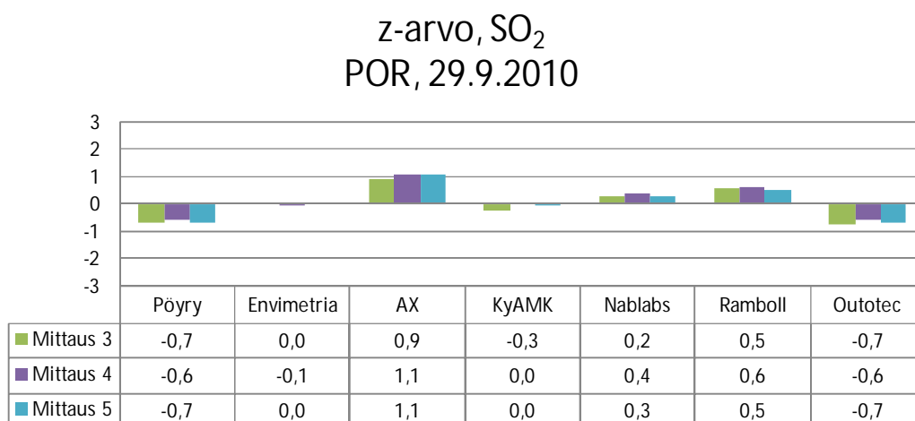
Kuva 9. z-arvot SO 2 -pitoisuustuloksille vertailumittauksissa 29.9.2010. Polttoaineena raskas polttoöljy POR.
