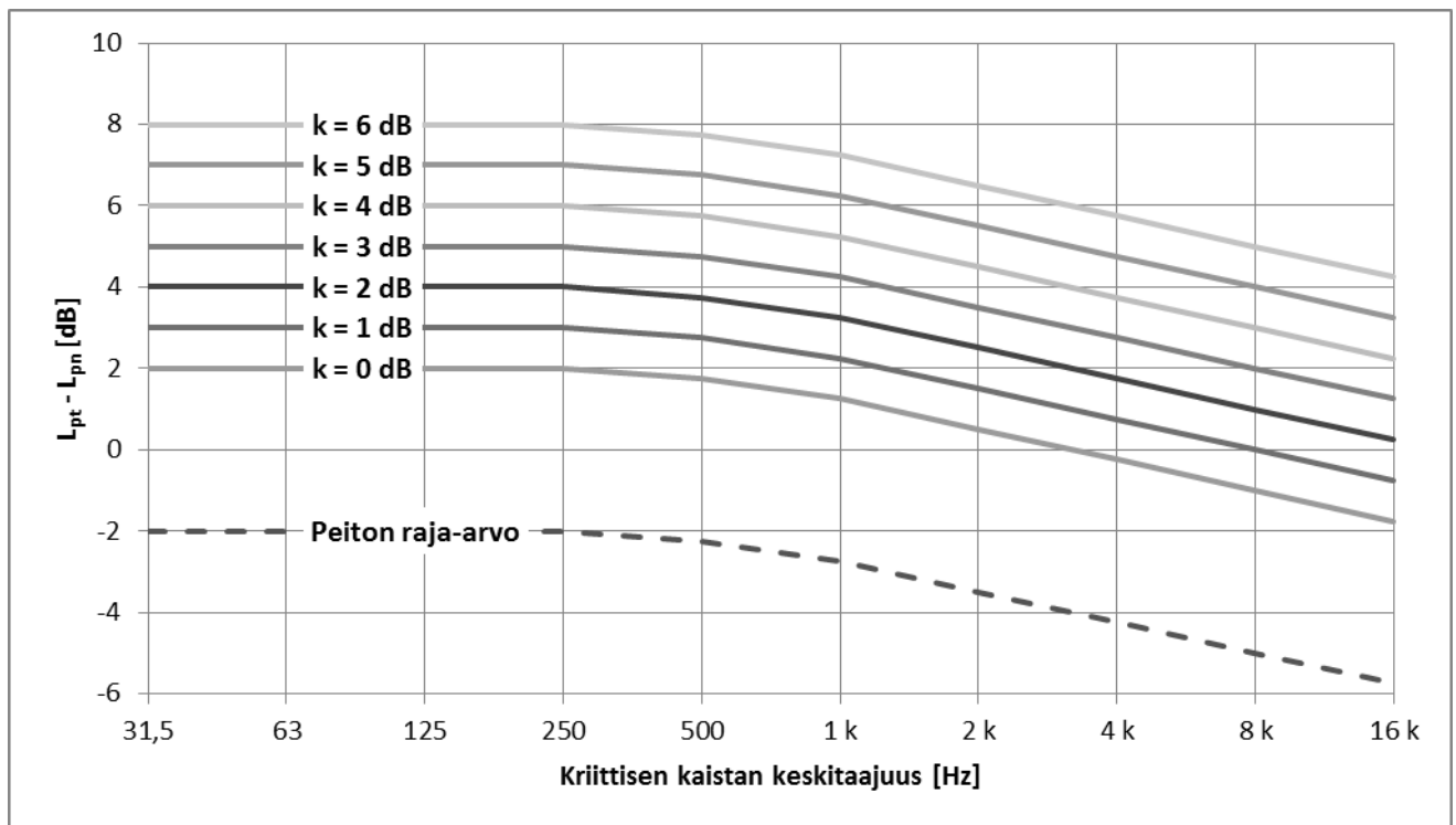
Kuva 5. Peittoäänien kynnysarvo ja käyrät sanktion k määrittämiseksi. L_{pt} on äänekseen tai kapeakaistaisen komponentin äänenpainetaso kriittisellä kaistalla, L_{pn} on peittoäänien äänenpainetaso samalla kriittisellä kaistalla. Kriittisen kaistan keskitaajuus ( f_c ) on vaakakselilla. (Pedersen et al., 2000)
