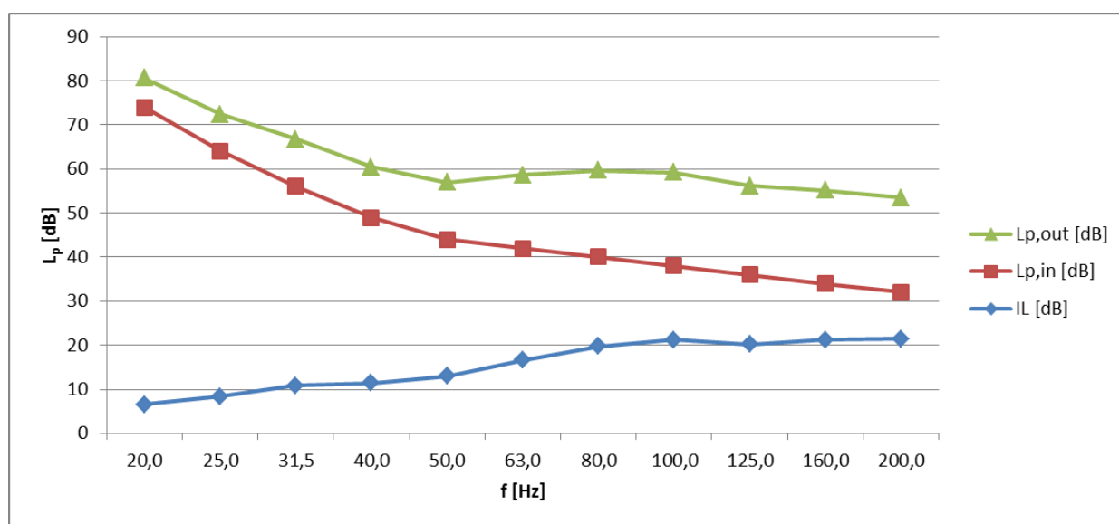
Kuva 8. Pienitaajuisten melun ohjearvot (vihreä kuvaaja, L_{p,out} ) rakennusten ulkopuolella perustuen asumisterveysohjeen ohjearvoihin (punainen kuvaaja, L_{p,in} ) ja tanskalaisten ääneneristysmääräyksiin (sininen kuvaaja, IL).
