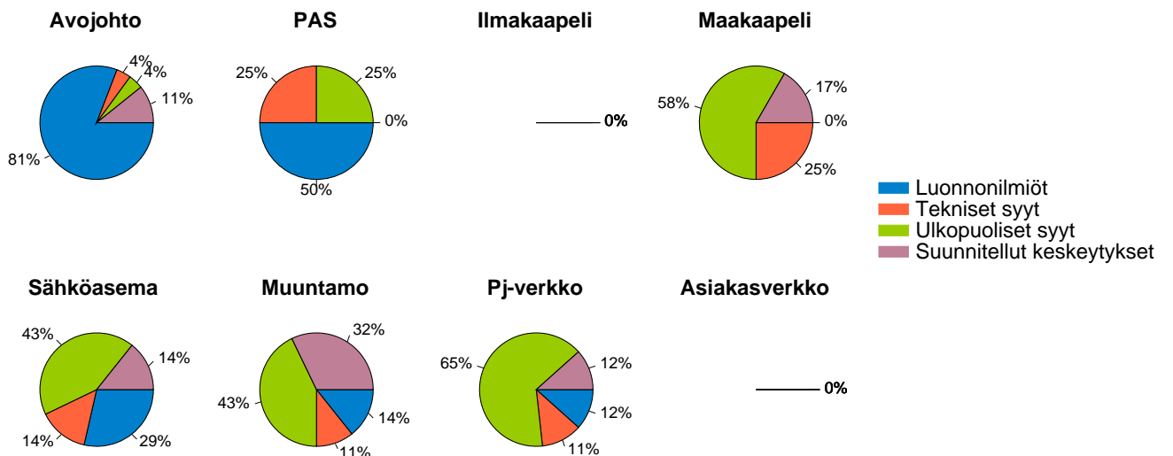
Eri verkon osien keskeytyksien aiheuttajat keskeytysajan suhteen
