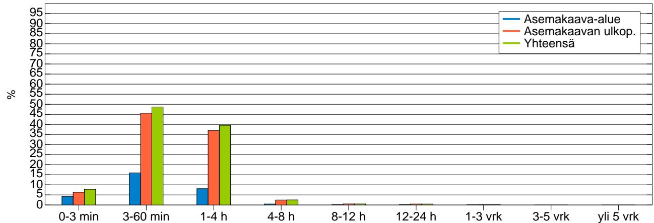
Keskeytysten jakauma keskipituuden (kph/kpk) mukaan (ei jälleenkytkentöjä)
