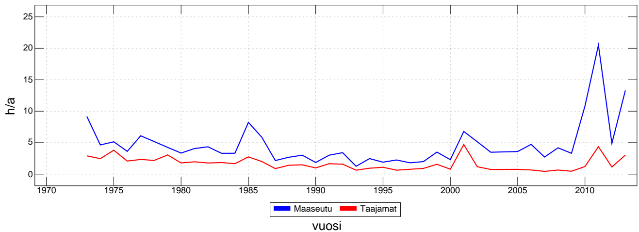
Asiakkaiden keskimääräinen häiriökeskeytysaika (h/a) vuosina 1973...2013
