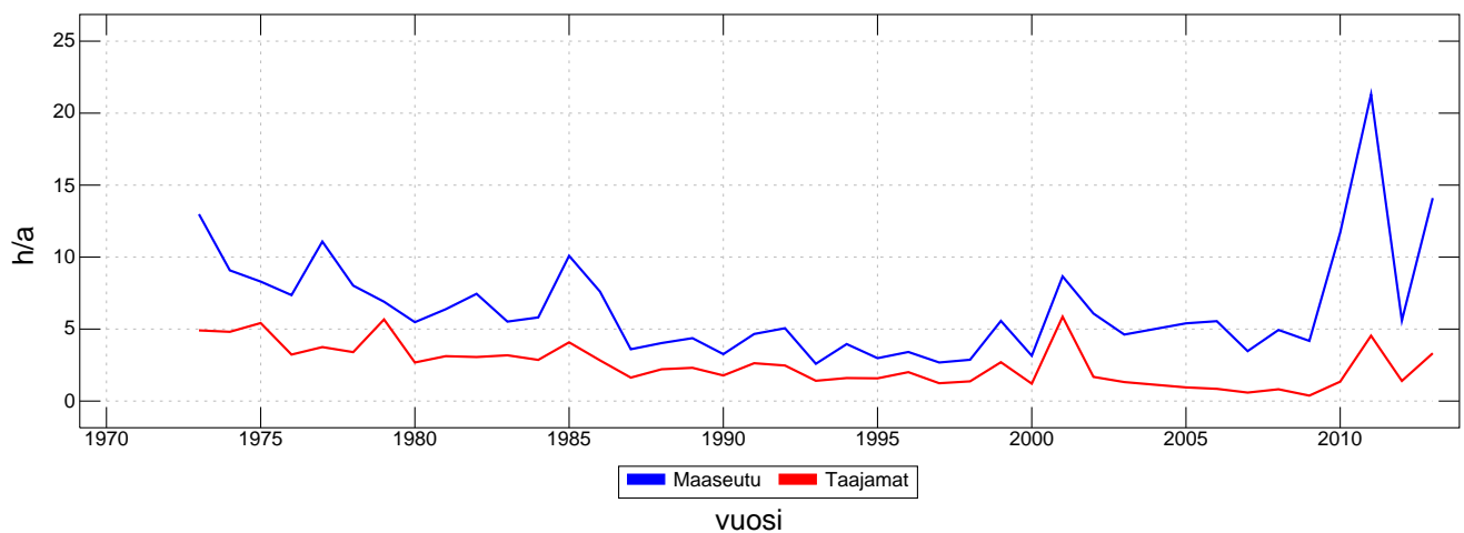
Keskeytyksistä asiakkaille aiheutunut sähkötön aika (h/a) vuosina 1973...2013
