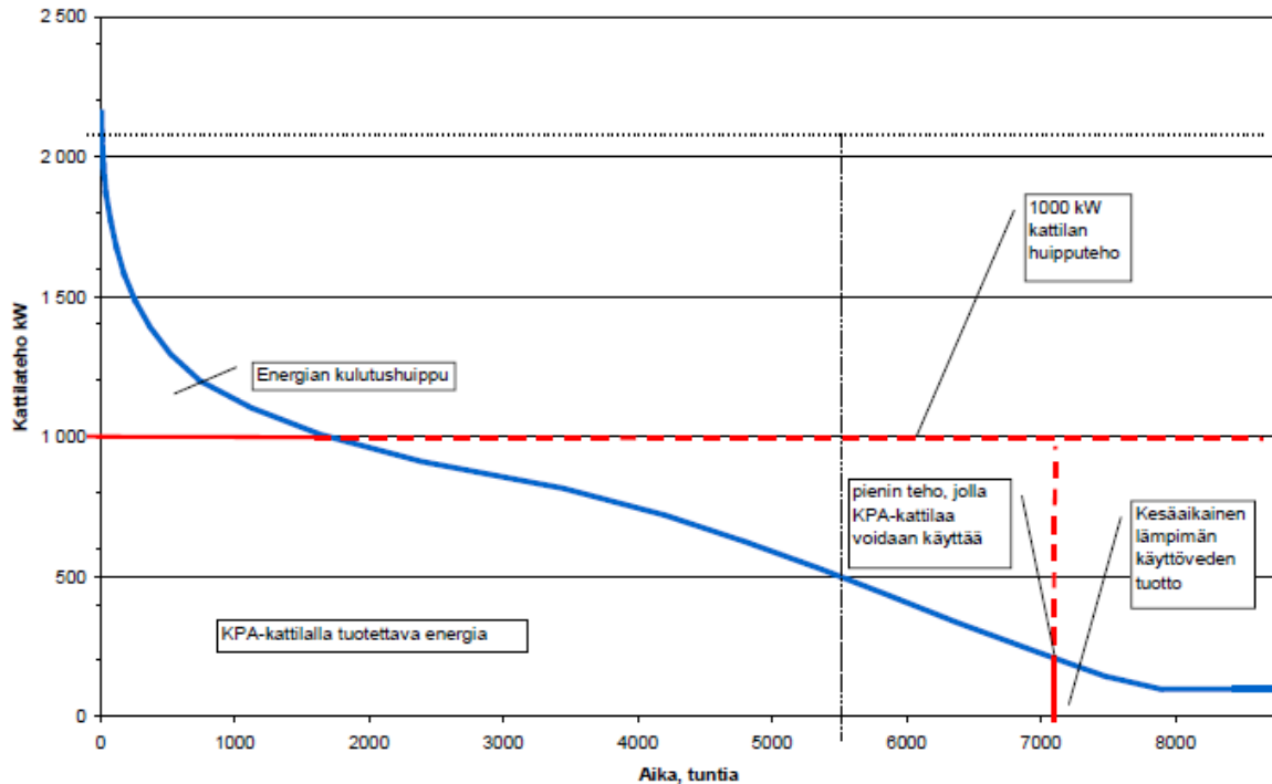
Kuva 12. Lämmitystehon pysyvyyskäyrä /10/.
